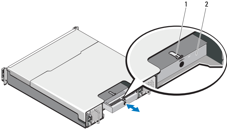
图 16-7. 卸下和安装 RAID 控制器模块挡片
